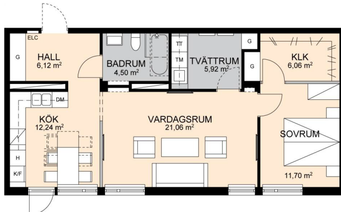
Figur 4.11: 2-3 RoK Alternativ 1 . Bostad för 1-2 personer.
