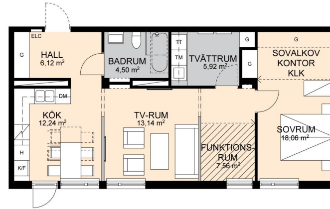
Figur 4.13: 2-3 RoK Alternativ 1 . Bostad för 1-4 personer.
